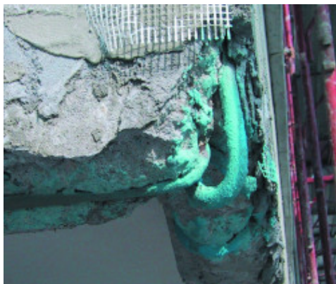
Mapefer 1K-val kezelt betonacélok az erkély homlokfelületén
